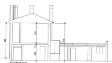
SEZIONE
